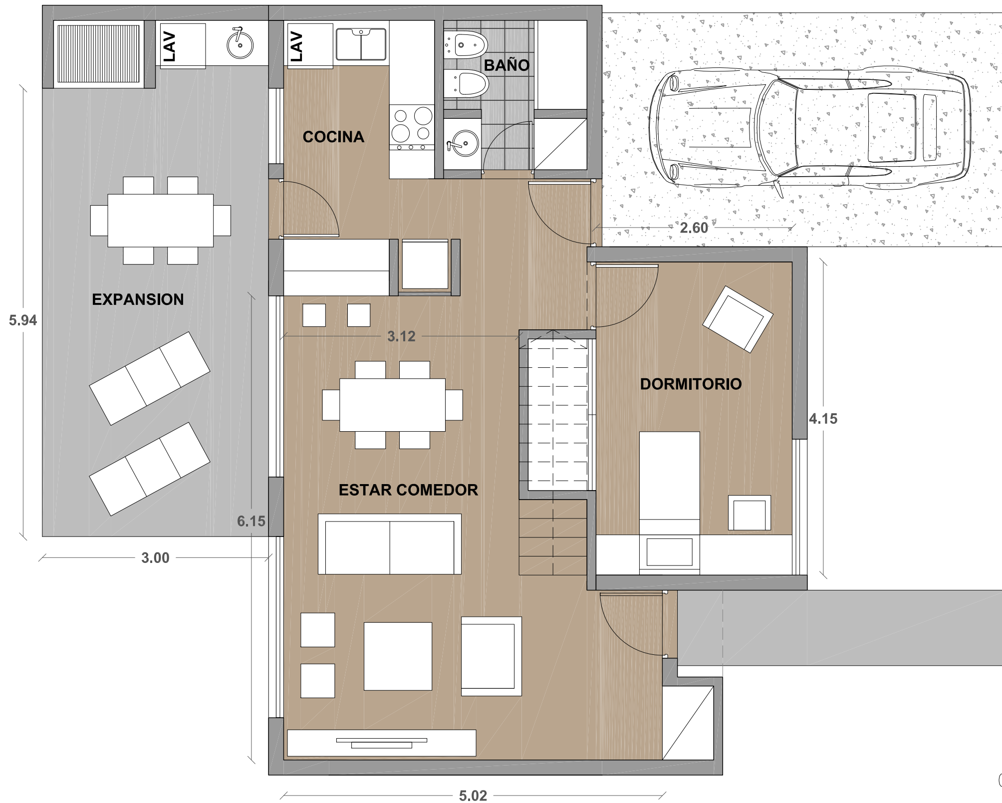
TIPOLOGIA C - planta baja
